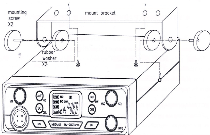
Рис.2. Пример крепления радиостанции при помощи монтажной скобы.
