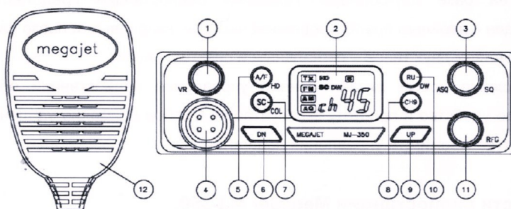
Рис. 1. Органы управления радиостанцией указаны цифрами.
