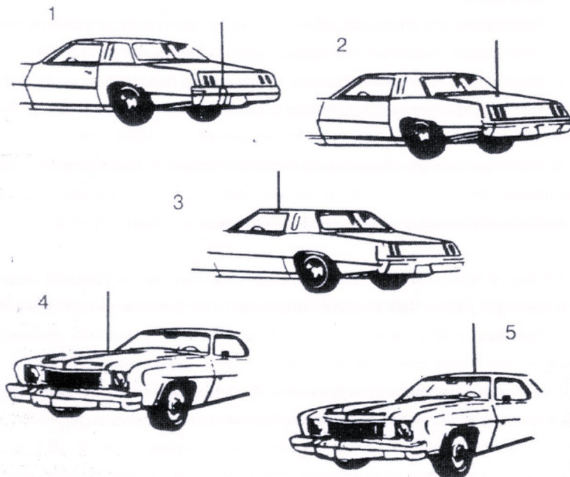
Рис. 6. Типичные места установки автомобильных антенн.
